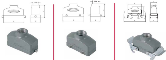
Size 24B «102x27» ⇒ A = 120.5 + B = 43.5 + C = 68 + F = 174 + L = 54
