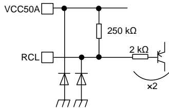
14) RCL pin
