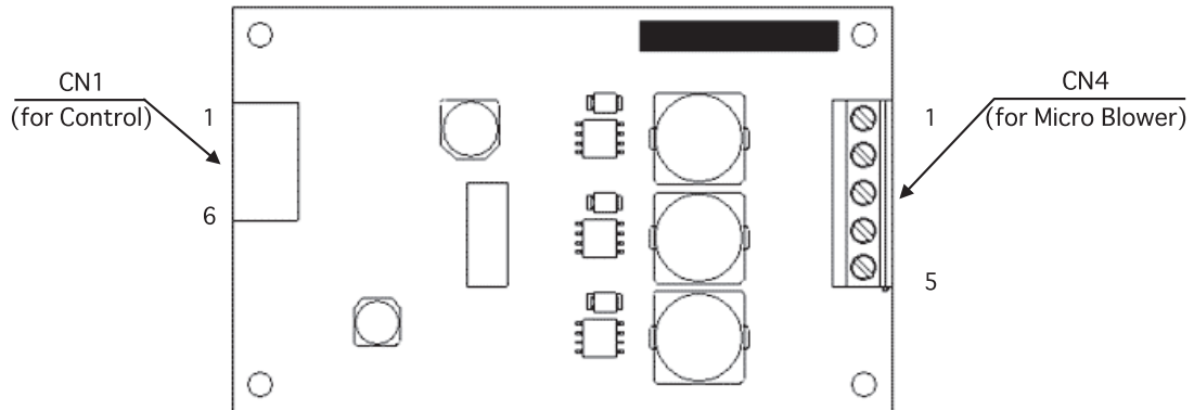
【Driver Board】
