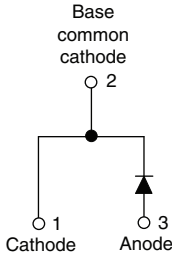
VS-60EPU06-N3
